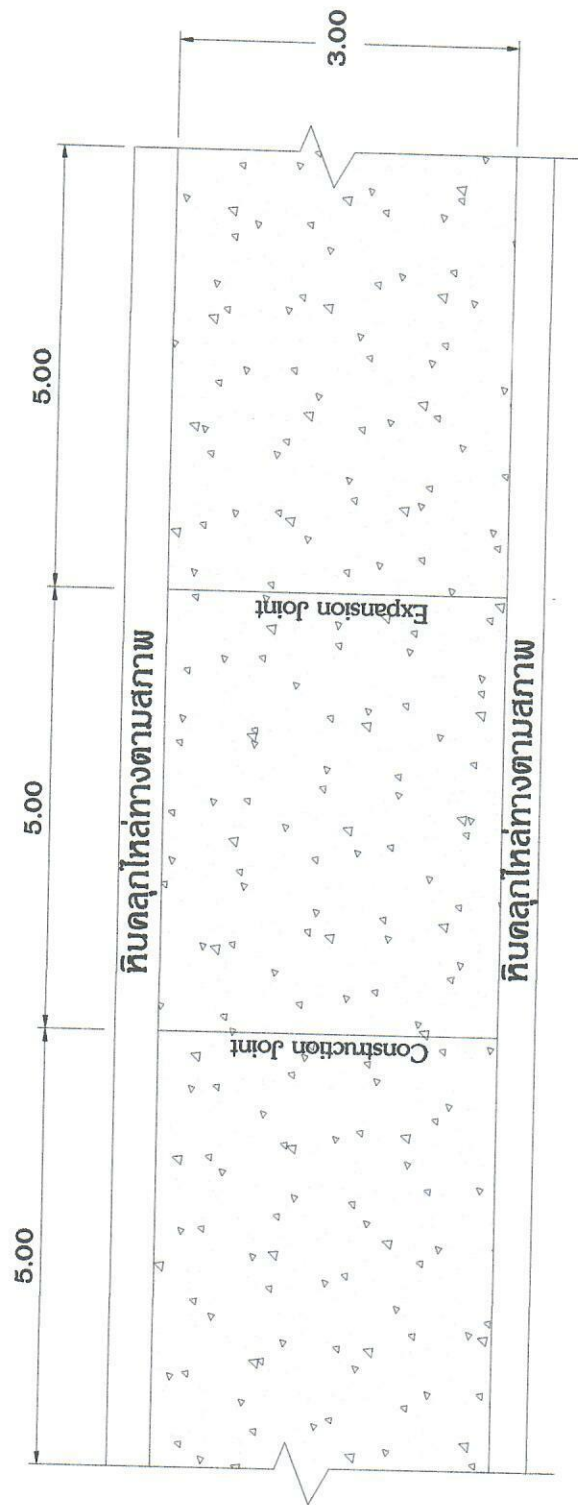
แปลนถนน คสล.
